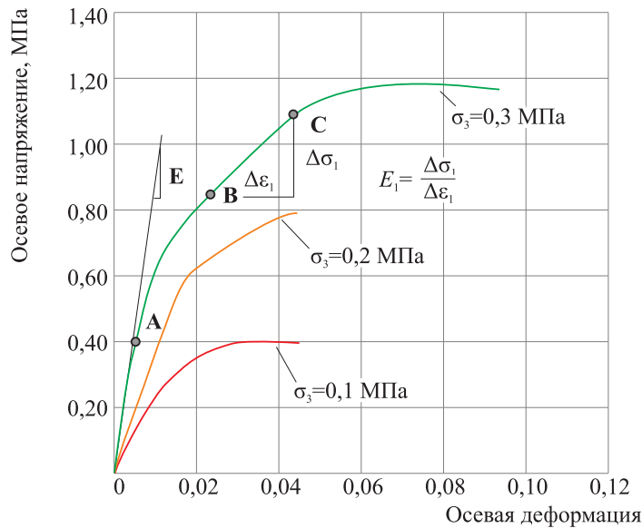
Рис. 2. Результаты испытаний в условиях трехосного сжатия: \sigma_3 — боковое давление; E — начальный модуль деформации; E_1 — секущий модуль деформации; \Delta\varepsilon_1 — приращение осевой деформации; \Delta\sigma_1 — приращение осевого напряжения
