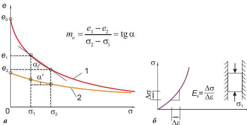
Рис. 8. К определению компрессионного (а) и одометрического (б) модулей деформации по данным испытаний в условиях компрессионного сжатия: 1 — ветвь первичного нагружения; 2 — ветвь разгрузки
