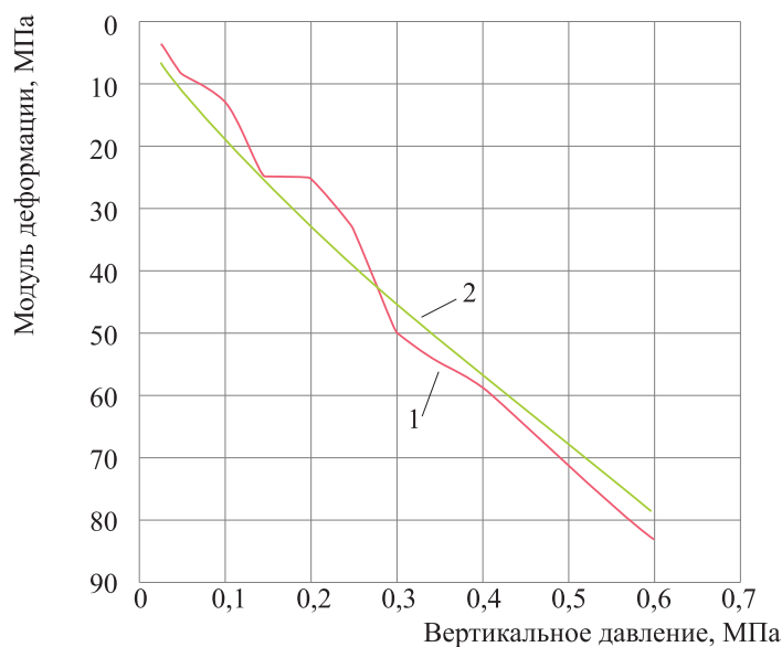
Рис. 5. Одометрические модули деформации: 1 — полученный по лабораторным данным; 2 — вычисленный по формуле (3)
