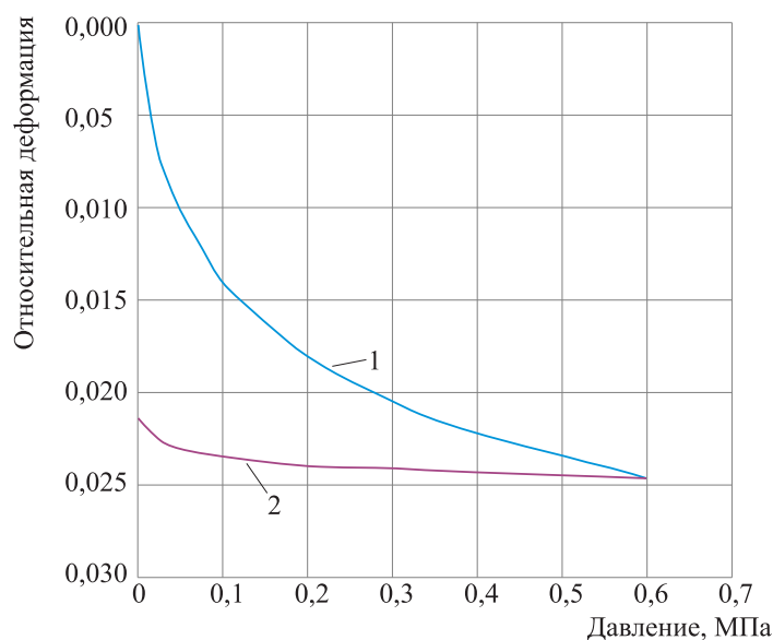
Рис. 3. Результаты испытаний в условиях компрессионного сжатия: 1 — ветвь первичного нагружения, 2 — ветвь разгрузки
