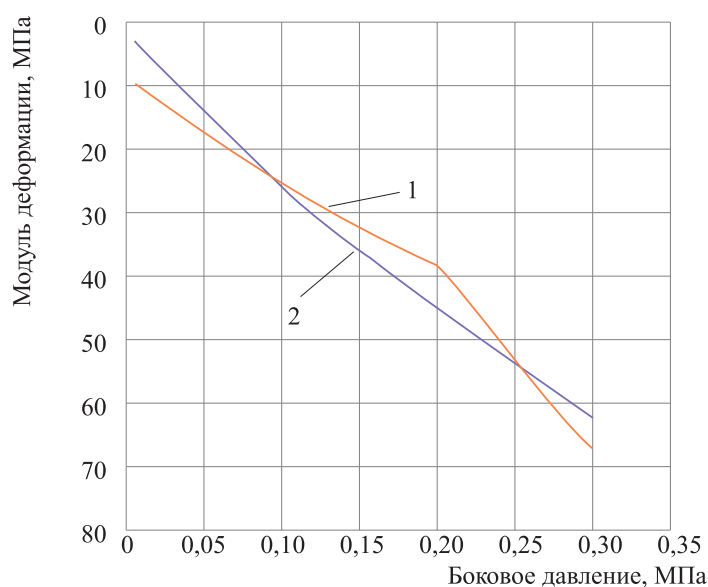
Рис. 4. Трехосные модули деформации: 1 — полученный по лабораторным данным; 2 — вычисленный по формуле (2)
