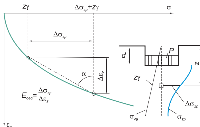
Рис. 9. К определению одометрического модуля деформации
