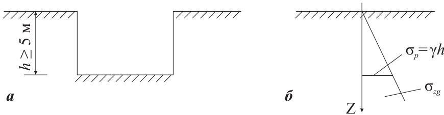
Рис. 7. К определению напряжений разгрузки: а — котлован в разрезе; б — эпюра напряжений \sigma_{zg} от собственного веса грунта; \sigma_{zg} = \sigma_{раз} — напряжение от веса грунта, удаленного при разработке котлована; h — глубина котлована; \gamma — удельный вес грунта (при наличии грунтовых вод находится с учетом взвешивающего действия воды)
