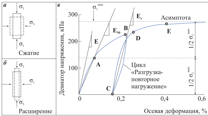
Рис. 6. К определению модулей деформации в условиях трехосного сжатия: а — траектория сжатия; б — траектория расширения; в — зависимость деформации от напряжения
