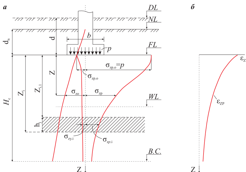
Рис. 1. Расчетная схема к определению осадки фундамента (а) и эпюра относительной вертикальной деформации \epsilon_z (б): d — глубина заложения подошвы фундамента; b — ширина фундамента; p — давление под подошвой фундамента; H_c — глубина сжимаемой толщи; DL — высотная отметка поверхности земли (природного рельефа); NL — отметка планировки; FL — отметка подошвы фундамента; WL — отметка уровня грунтовых вод; В.С. — нижняя граница сжимаемой толщи
